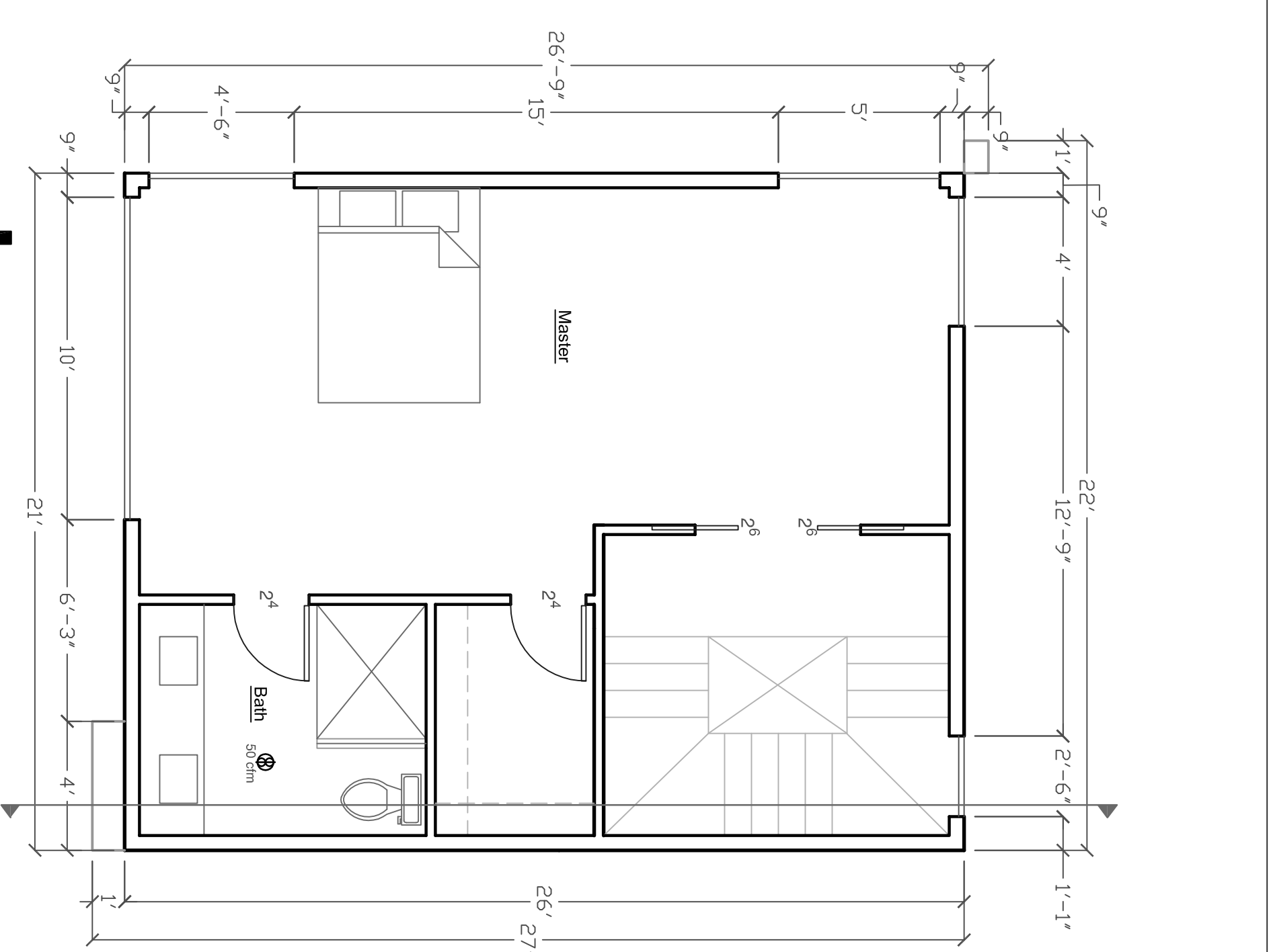
UPPER SCALE: 1/4" = 1'-0"
