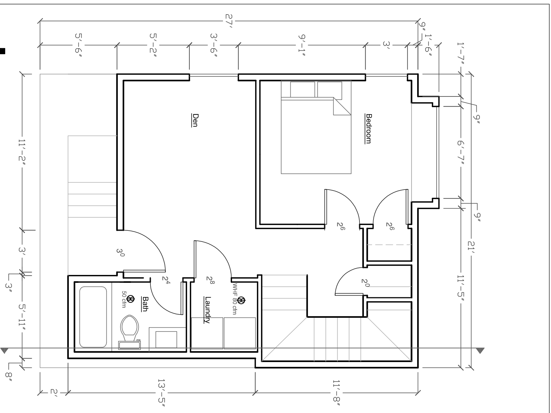
LOWER SCALE: 1/4" = 1'-0"
